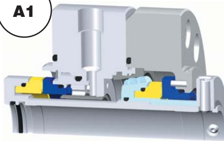
План API 54 (опция)
