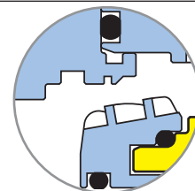
План API 54 (опция)
