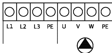
Схема подключения (3~400 В)
