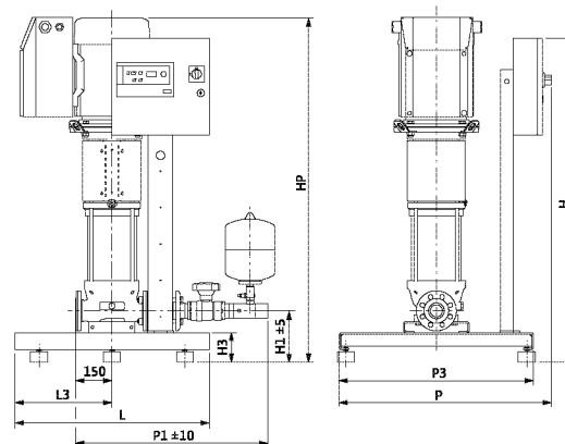
Габаритный чертеж
