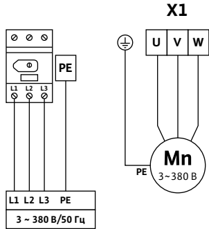
Схема подключения SK 712-ss
