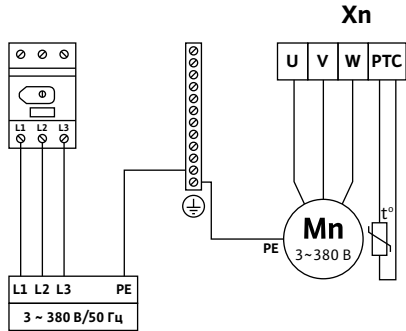
Схема подключения SK 712-sd
