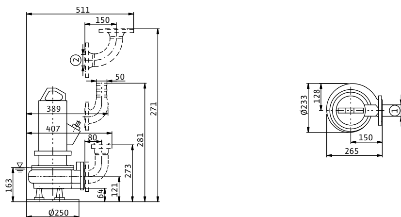
Чертеж с размерами Wilo-EMU FA...RF – мобильная установка
