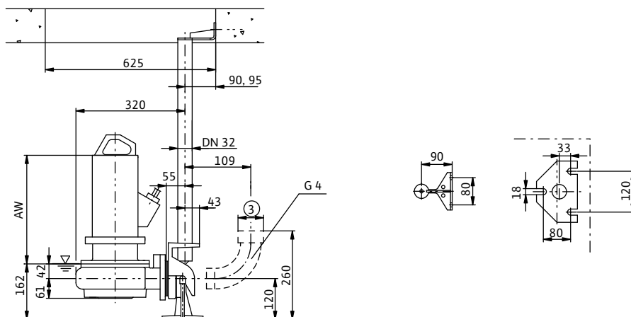
Чертеж с размерами Wilo-EMU FA...RF – стационарная погружная установка
