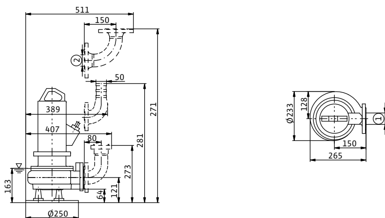
Чертеж с размерами Wilo-EMU FA...RF – мобильная установка
