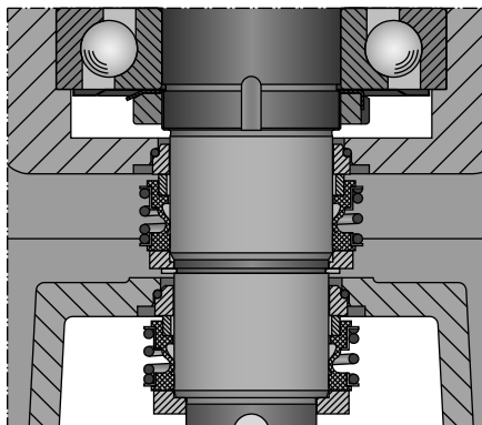
Изображение: два СТУ в тандемной установке для тяжелых условий эксплуатации
