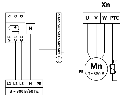
Схема подключения SK 712-d
